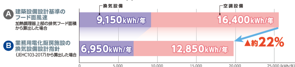
図 1-2 本指針と建築設備設計基準(排気フード面風速からの算出)での換気量と消費電力量比較
